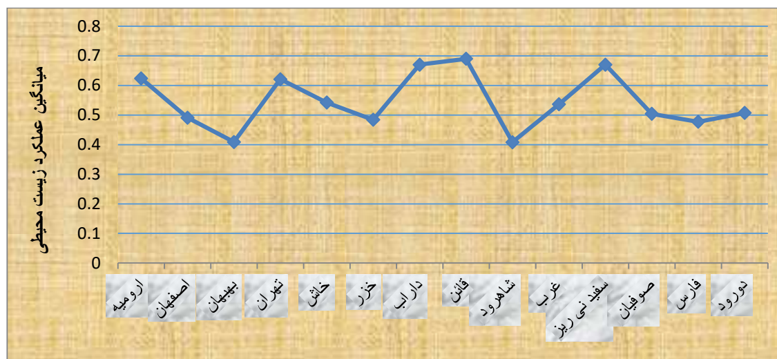
شکل ۱- میانگین عملکرد زیست محیطی شرکت‌های سیمان طی ۱۳۸۷ تا ۱۳۹۶
