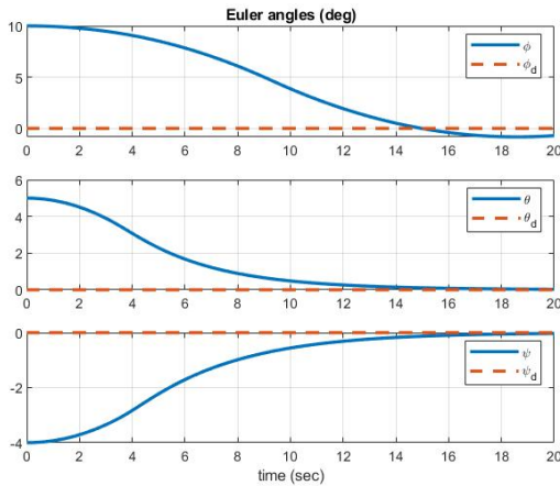
شکل ۸- زوایای اوپلر در حالت دوم
