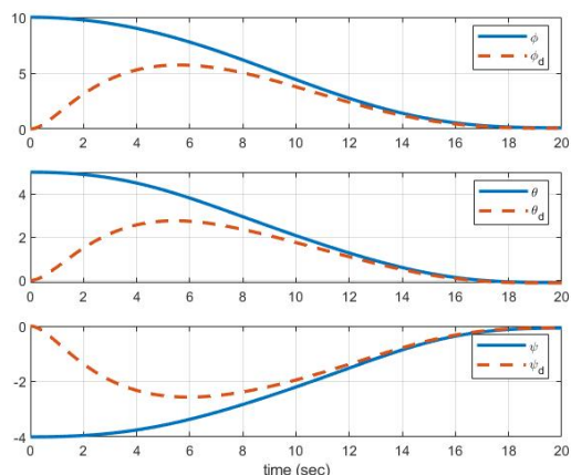
شکل ۱۱- زوایای اوایلر در حالت سوم
