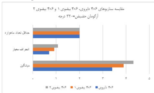
شکل ۵. مقایسه سناریوهای تک‌منتظم (4x6): ( \Omega=320 و e=0,0.19,0.097 )
