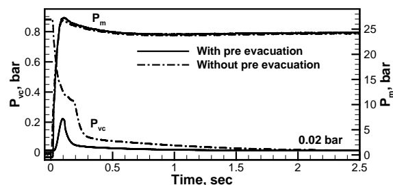
شکل ۷- مقایسه مدت زمان راه اندازی در حالت بارگذاری آبی بدون پیش خلاءسازی و همراه با پیش خلاءسازی در نسبت سطح ۱/۸
