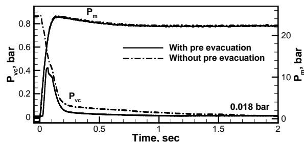
شکل ۶. مقایسه مدت زمان راه اندازی در حالت بارگذاری آبی بدون پیش خلاءسازی و همراه با پیش خلاءسازی در نسبت سطح ۱/۷
