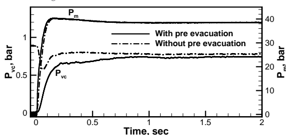
شکل ۹. مقایسه مدت زمان راه اندازی در حالت بارگذاری آبی بدون پیش خلاءسازی و همراه با پیش خلاءسازی در نسبت سطح ۱/۹
