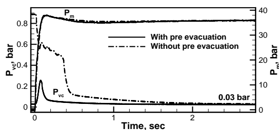
شکل ۸- مقایسه مدت زمان راه اندازی در حالت بارگذاری آبی بدون پیش خلاءسازی و همراه با پیش خلاءسازی در نسبت سطح ۱/۸۵
