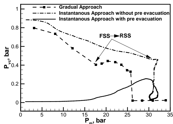
شکل ۱۳. فشار محفظه خلاء بر حسب فشار محفظه نازل در بارگذاری های تدریجی، آنی همراه و بدون پیش خلاءسازی در نسبت سطح ۱/۸
