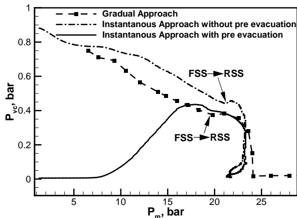
شکل ۱۲. فشار محفظه خلاء بر حسب فشار محفظه نازل در بارگذاری های تدریجی، آنی همراه و بدون پیش خلاءسازی در نسبت سطح ۱/۷
