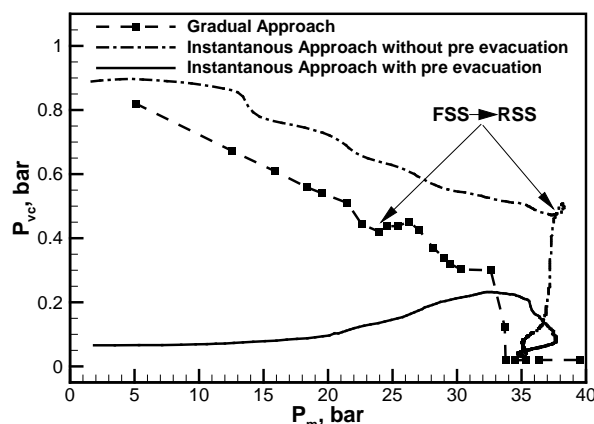
شکل ۱۴. فشار محفظه خلاء بر حسب فشار محفظه نازل در بارگذاری‌های تدریجی، آبی همراه و بدون پیش خلاءسازی در نسبت سطح ۱/۸۵
