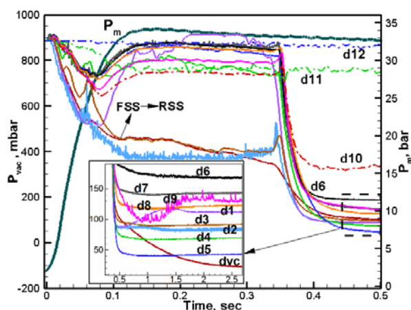
شکل ۱۵. نمودار فشار لحظه‌ای تمامی سنسورهای بستر آزمون در بارگذاری آبی و بدون پیش خلاءسازی ( P_{m,ave}=31.2 \text{ bar} )
