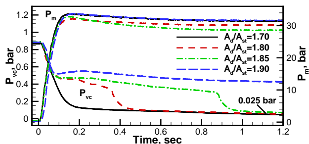
شکل ۵. فشار محفظه نازل و محفظه خلأ بر حسب زمان در حالت بارگذاری آبی بدون پیش‌خلأ‌سازی و در نسبت‌های مختلف
