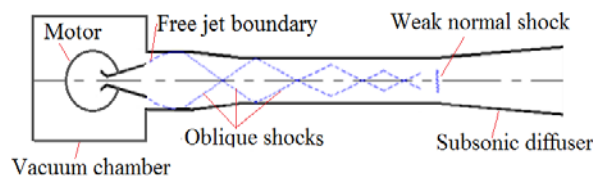
شکل ۱. شماتیکی از هسته مرکزی بستر شبیه‌ساز ارتفاع بالا و جریان داخل آن
