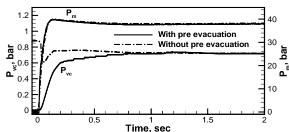
شکل ۱۰. مقایسه مدت زمان راه اندازی در حالت بارگذاری آبی بدون پیش خلاءسازی و همراه با پیش خلاءسازی در نسبت سطح ۲
