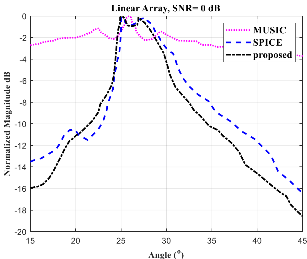
شکل ۵: تابع جستجوی نرمالیزه شده الگوریتم‌های طبقه‌بندی سیگنال چندگانه، SPICE و پیشنهادی اول برای آشکارسازی هدف در SNR=0dB
