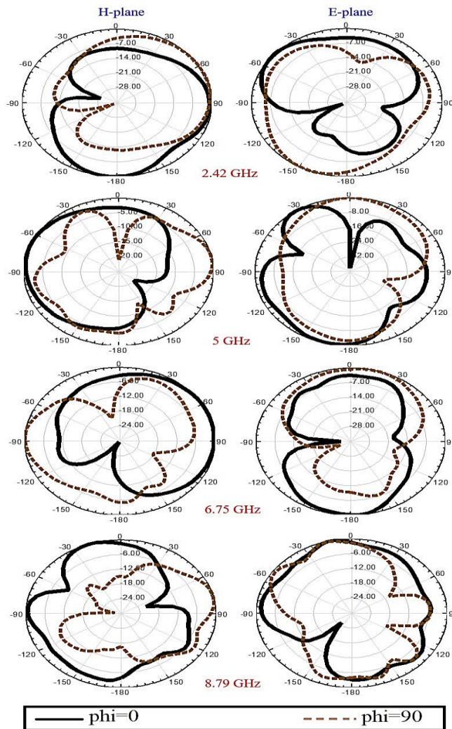
شکل ۱۱: پترن تشعشی E-plane و H-plane آنتن پیشنهادی در فرکانس‌های رزونانس
