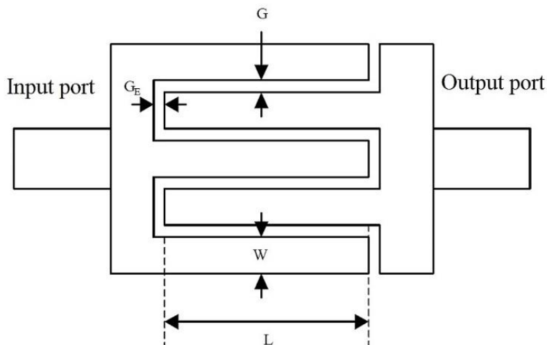
شکل ۱: ساختار خازن بین انگشتی (IDC)
