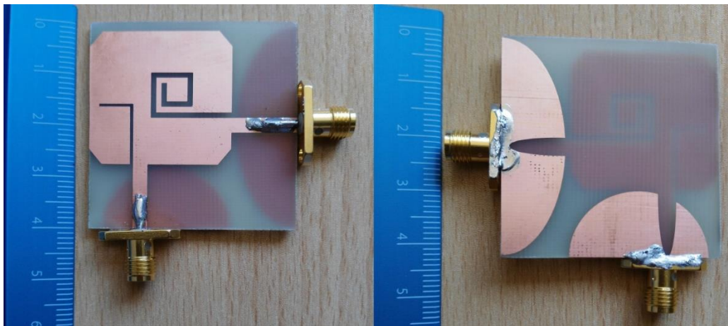
شکل ۱۱: عکس نمونه تشعشع کننده محقق شده نتیجه گیری
