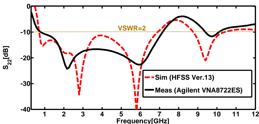
شکل ۳: منحنی شبیه‌سازی شده و سائزگیری شده افت برگشتی برای دهانه دو ( S_{22} )
