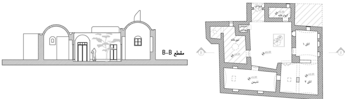
ت ۱۵. پلان و مقطع نمونه یک - خانه رقیه قاسمی، روستای خور، فاز صفر پروژه طراحی خانه در خور.
