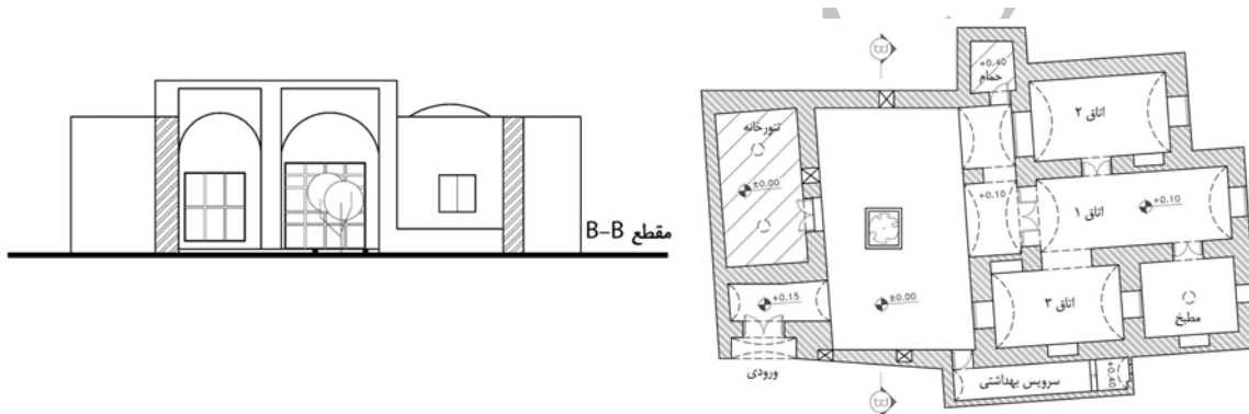
ت ۱۶. پلان و مقطع نمونه دو - خانه رضا شاهوردی، روستای خور، فاز صفر پروژه طراحی خانه در خور.
