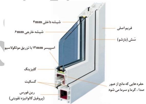
ت ۱۵. نمونه‌ای از یک قاب UPVC.
