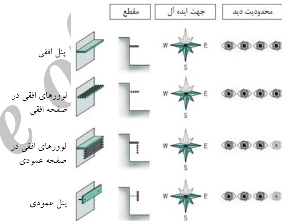
ت ۷. انواع سایبان افقی.
