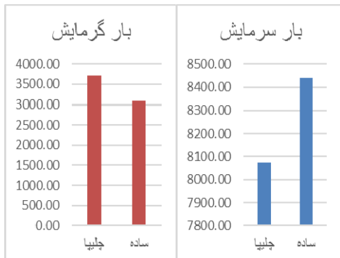
ن ۲. بار سرمایش بر حسب کیلو وات ساعت در خانه دهقان در فرم چلیپا و مستطیل.
