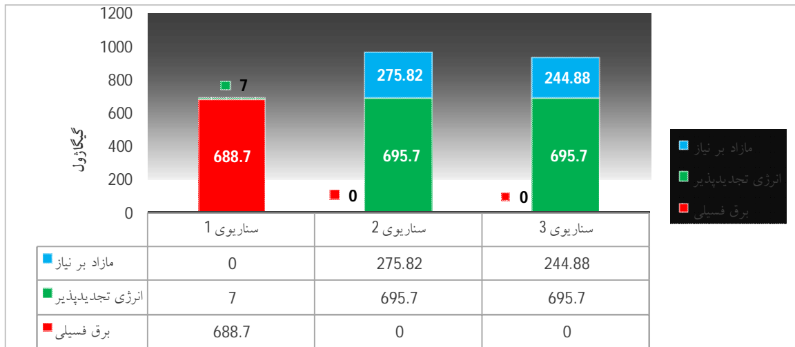
ن 5. نسبت تشکیل‌دهنده برق تولیدی و مصرفی روستای نجوهران در یک سال بر حسب نوع منبع تولید.
