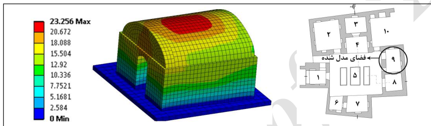
ت 5. مدل‌سازی و نمایش حداکثر تغییر شکل سازه در حالت تقویت نشده (نگارندگان، 1395).
