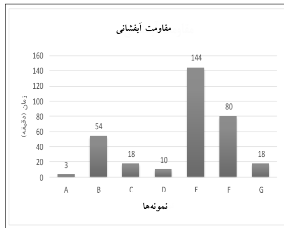
ن ۳. نمودار مقاومت آبشانی آزمونه‌ها، منبع: نگارندگان.
