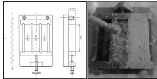
ت ۲. قالب ۴۰*۴۰*۱۶۰ (ابعاد برحسب میلی‌متر) استفاده شده جهت انجام آزمون خمشی، منبع: نگارندگان.
