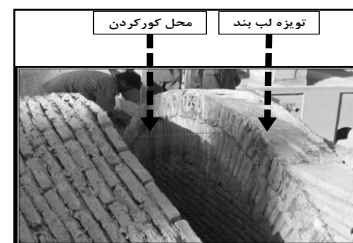
ت ۱۱. کور کردن تاق لی لی پوش یک سویه (منبع: نگارندگان، شهر ابرکوه استان یزد).
