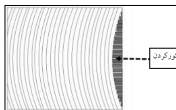
ت ۱۰. پلان و نمایی از تاق لی لی پوش دوسویه (کشیده) (منبع: نگارندگان).
