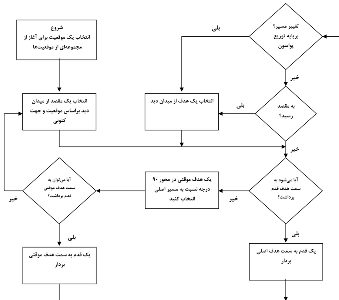
نمودار ۱: روند تصمیم‌گیری کاربر در مدل EVA
