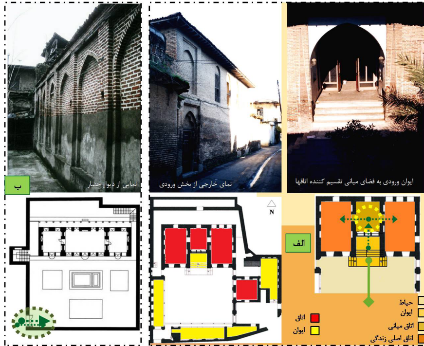
شکل ۹: مقایسه ورودی دو خانه از طبقه متوسط در گیلان و مازندران. الف- ورودی غیرمستقیم در خانه باباپور، بابل، مازندران (نمونه‌ای از خانه درونگرا) ب- ورودی منفصل خانه اشکوری در رشت
