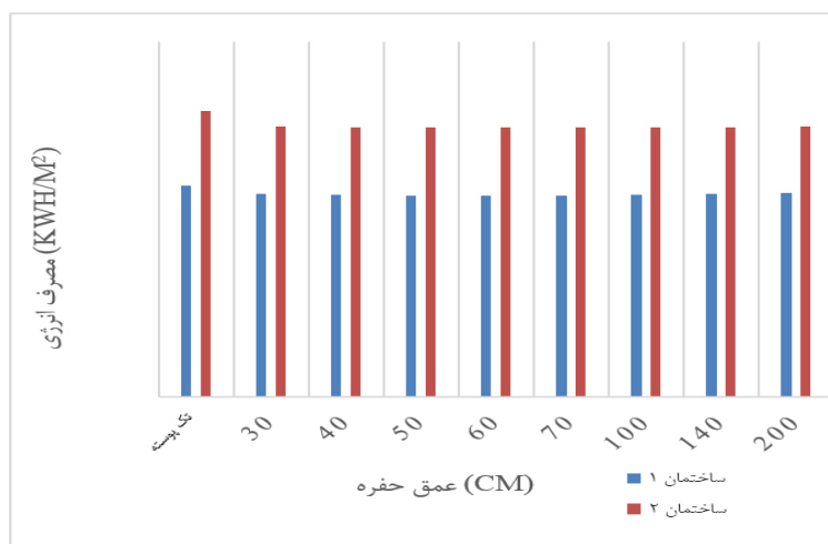
شکل ۸: میزان مصرف انرژی سرمایشی در ساختمان‌های ۱ و ۲
