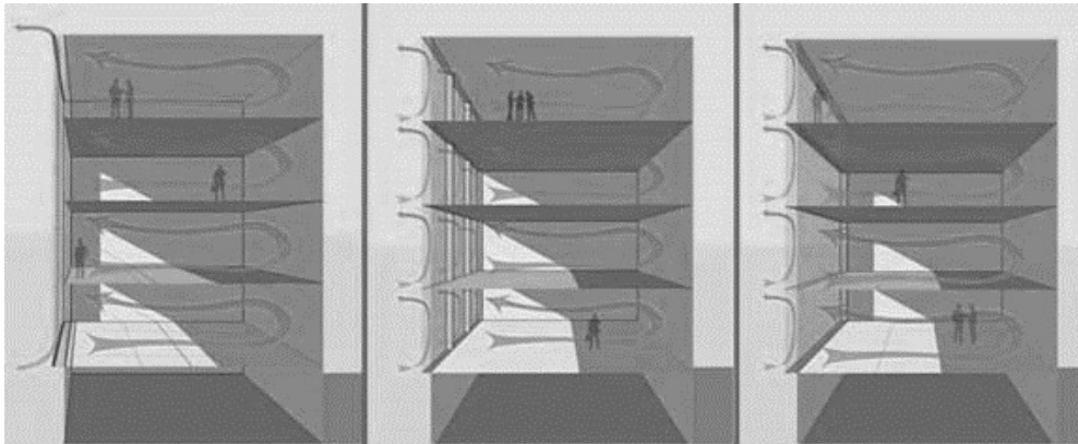
شکل ۱۷: نمودار تهویه طبیعی گونه‌های مختلف نمای دوپوسته در تابستان (دریچه‌ها تابستان: روشن - زمستان: خاموش)
