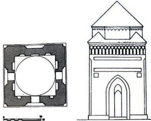
تصویر ۶. نقشه مقبره شمس آل رسول (ویلبر، ۱۳۷۵: ۹۹۵)
