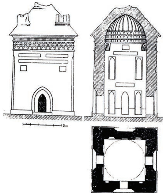
تصویر ۳. نقشه های مقبره های شمس آل رسول از ترسیمات دمرگان (ستوده، ۱۳۶۶)
