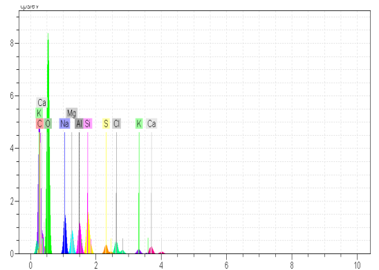
تصویر ۴-الف. تجزیه عنصری پوست به روش EDX (نگارندگان).
