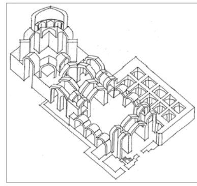
تصویر ۱۰. درهم تنیدگی کالبدی اجزای سازه‌ای مجموعه (نگارندگان)
