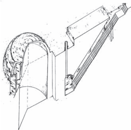
نگاره ۱: اندام یک آب‌انبار در نقاط مرکزی ایران شامل مخزن و پوشش، پاشیر، پلکان و بادگیر. (مأخذ: معماریان، ۱۳۸۷)
