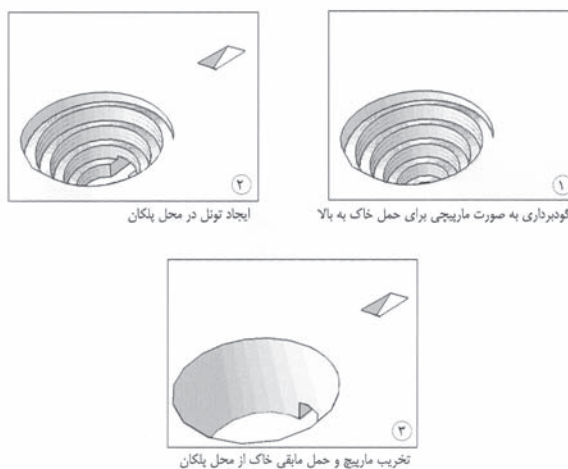
مراحل ساخت آب‌انبار (خاکبرداری)
