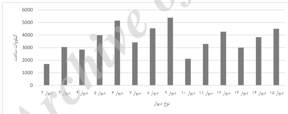
شکل ۶. کاهش متوسط مصرف انرژی سالیانه جهت سرمایش و گرمایش نسبت به دیوار پایه (دیوار ۱) بر حسب کیلو وات ساعت
