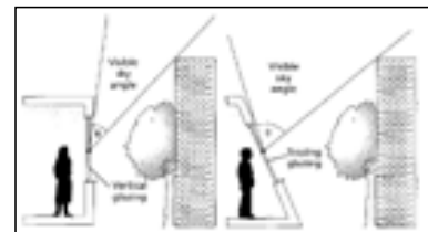
تصویر ۷- روش تعیین زاویه دید آسمان از نورگیر (Ref: Lighting Guide ۱۰, ۱۹۹۹, p. ۲۵)
