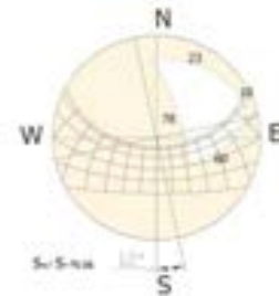
تصویر ۷- روش تعیین زاویه دید آسمان از نورگیر (Ref: Lighting Guide ۱۰, ۱۹۹۹, p. ۲۵)
