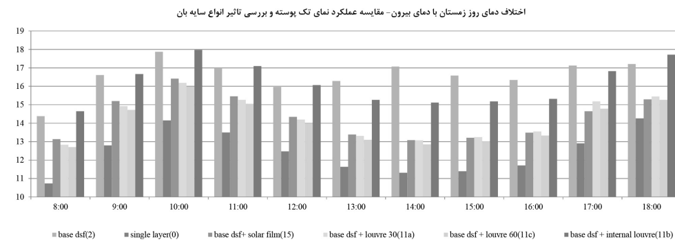
تصویر ۷: دمای روز زمستانی، مقایسه عملکرد نمای تک پوسته و بررسی تأثیر انواع سایبان در محدوده ساعات تصرف فضا
