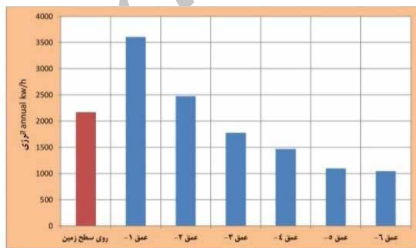
نمودار ۵: مصرف سالانه انرژی گرمایشی در اعماق ۱- متری تا ۶- متری در مقایسه با مدل مشابه روی زمین در شهر تهران
