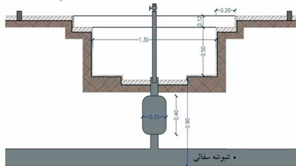
تصویر ۲۲: برش حوض ستاره‌ای که در آن، طرز کار فواره‌های باغ مشخص شده است.
