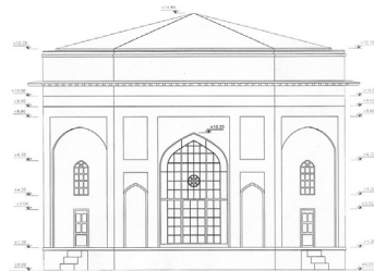
نمای شرقی
