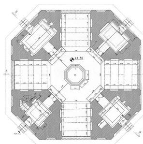
پلان همکف
