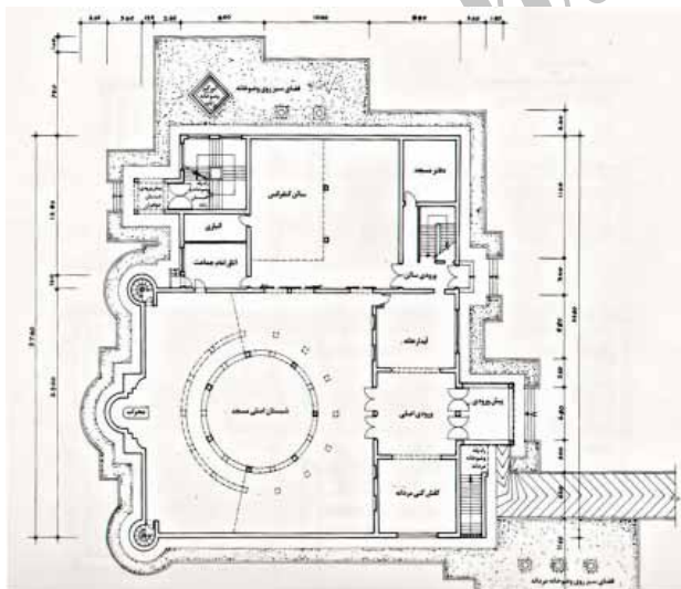
تصویر ۳. پلان طبقه همکف مسجد بلال (مأخذ: زم‌رشیدی ۱۳۷۴، ۳۳۸)
