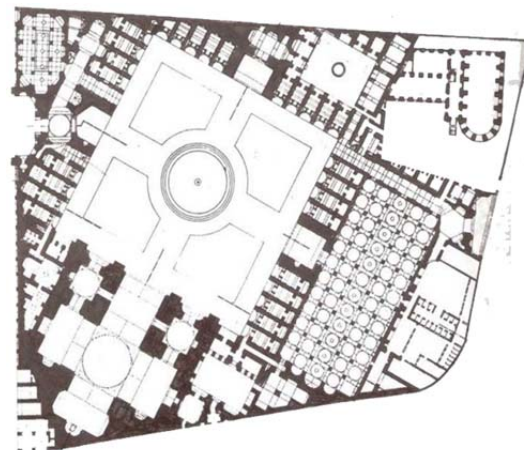
شکل ۶) پلان وضع موجود مسجد- مدرسه؛ ماخذ: آرشیو کتابخانه مسجد- مدرسه سپهسالار
