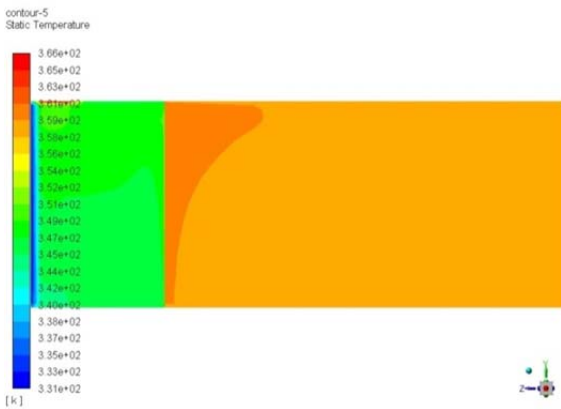
شکل (۷) کانتور دما در مقطع عرضی حالت پنجم
