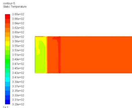
شکل (۱۰) کانتور دما در مقطع عرضی حالت دوم
