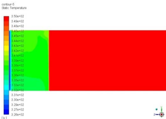
شکل (۹) کانتور دما در مقطع عرضی حالت ششم
