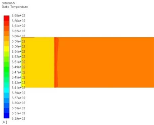
شکل (۵) کانتور دما در مقطع عرضی حالت سوم
