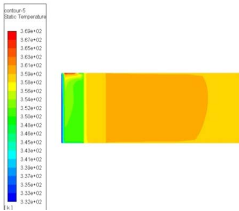
شکل (۶) کانتور دما در مقطع عرضی حالت چهارم
