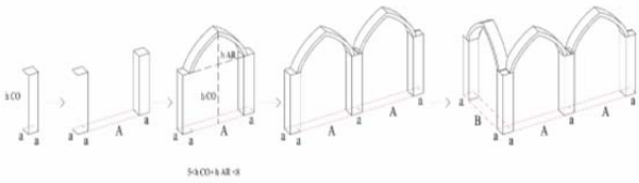
شکل ۱۰) قسمتی از فرآیند ساخت مدول‌های کارخانه با سیستم سنتی تاق و تویزه (منبع: نویسندگان)
