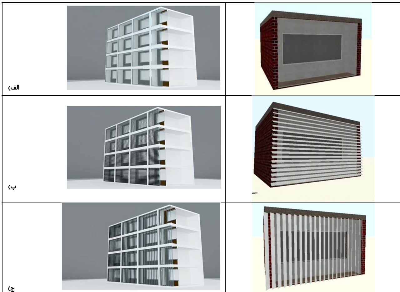
شکل (۶) مدل اتاق اداری با نمای دوپوسته: الف) بدون سایه‌انداز، ب) سایه‌اندازهای کرکره‌ای افقی، ج) سایه‌اندازهای کرکره‌ای قائم
