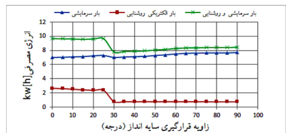
نمودار (۳) میزان مصرف انرژی در ۵ آگوست با لور افقی
