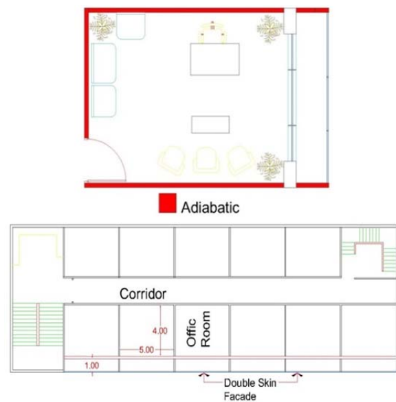
شکل ۲) پلان مجموعه اداری (بالا)؛ پلان یکی از اتاق‌های اداری به همراه نواحی آدیباتیک (پایین)
