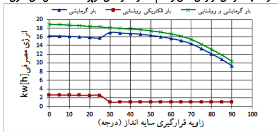
نمودار (۴) میزان مصرف انرژی در ۲۱ ژانویه با لور افقی
