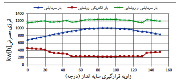
نمودار (۲) میزان مصرف انرژی سالیانه با لورهای افقی قائم
