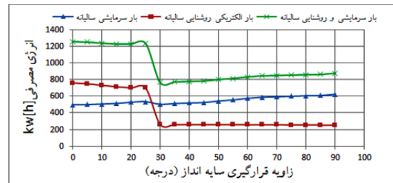
نمودار (۱) میزان مصرف انرژی سالیانه با لورهای افقی ثابت
