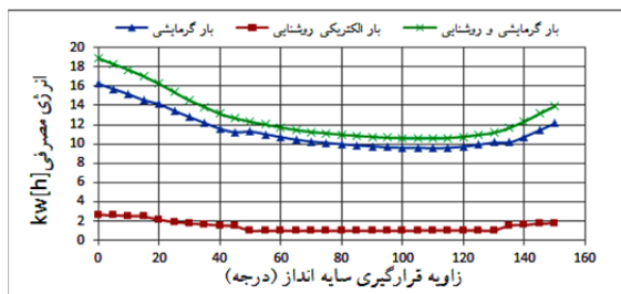
نمودار (۶) میزان مصرف انرژی در ۲۱ ژانویه با لور قائم
