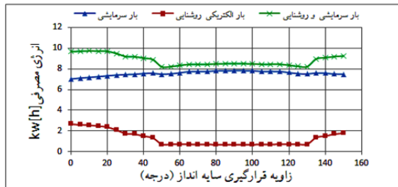
نمودار (۵) میزان مصرف انرژی در ۵ آگوست با لور قائم
