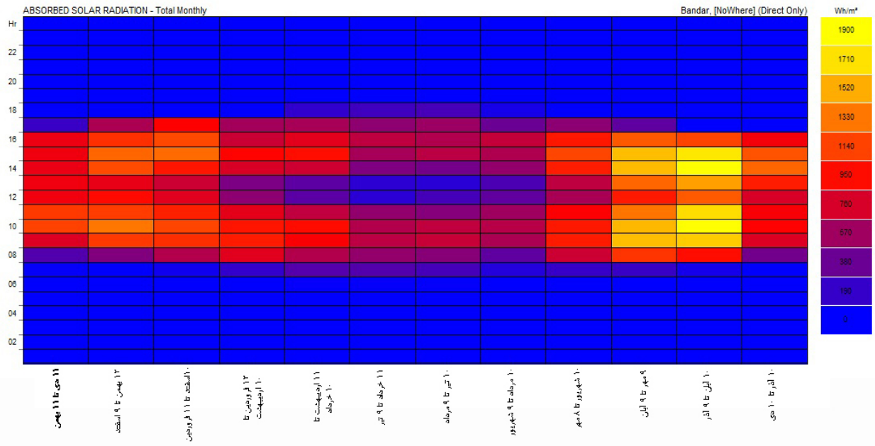
نمودار ۷) میانگین ماهانه انرژی تابشی دریافتی برای مدل CO-W-8
