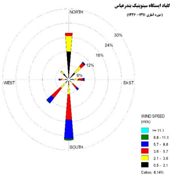
شکل ۳) کلیاد شهر بندرعباس برای بازه زمانی ۱۳۳۶ تا ۱۳۹۱؛ اداره کل هواشناسی استان هرمزگان [37]
