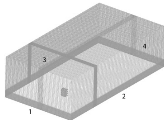
شکل ۲) شبکه‌بندی دامنه محاسباتی و شرایط مرزی؛ (۱) Velocity inlet، (۲) Symmetry، (۳) Symmetry، (۴) Pressure outlet
