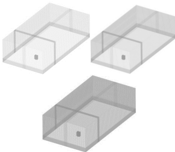
شکل ۴) دامنه مدل‌های محاسباتی با سه اندازه و تعداد مش متفاوت؛ ابعاد مش در ریزترین شبکه ۰/۱ و در درشت‌ترین حالت برابر با ۰/۶ است.
