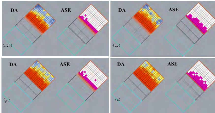
تصویر ۴- گراف کفایت نور روز و نفوذ سالیانه نور خورشید در جبهه شمالشرقی (خانه ابریشمی) (ماخذ:)
