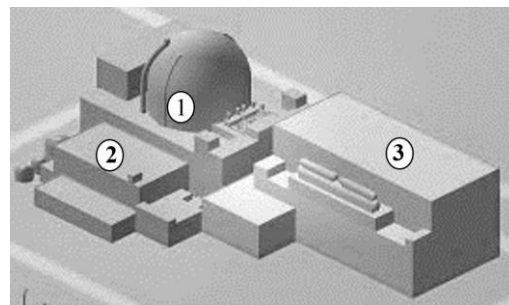
تصویر ۳: طرح شماتیک نیروگاه تحت فشار پیشرفته؛ (۱) ساختمان راکتور، (۲) ساختمان جانبی، (۳) ساختمان توربین؛ مأخذ: (Suzuki et al. 2009: 18)
