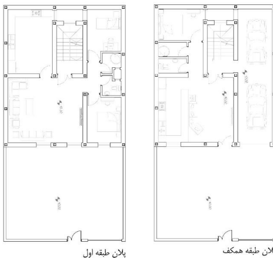
تصویر ۳- پلان طبقه هم کف و اول نمونه موردی (ابعاد زمین: ۱۰*۱۹/۵)
