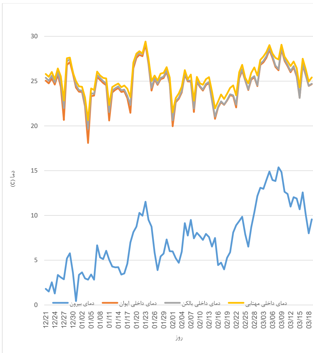
تصویر ۱۴- نمودار همبستگی دمایی فضای داخلی گلخانه‌ها و محیط بیرون در زمستان و با پوشش شیشه تک جداره (ماخذ:
