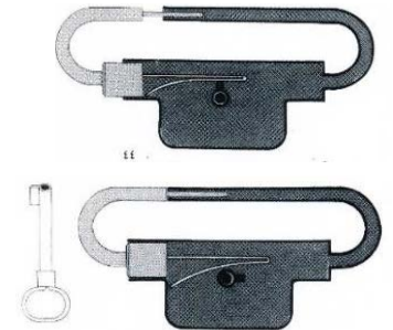
تصویر ۱۴: مکانیزم درونی فنر خاردار (تناولی، ۱۳۸۶، ۲۹).
