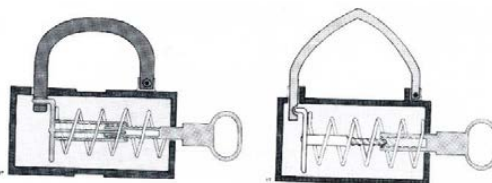
تصویر ۱۳: مکانیزم درونی قفل‌های چالستر با فنر ماریچ (تناولی ۱۳۸۶، ۳۳).
