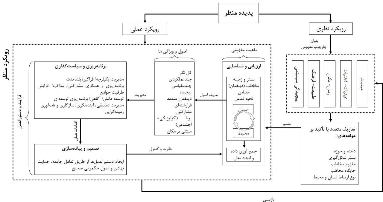
تصویر ۵. فرایند تحلیل مفهوم منظر و رویکرد منظر و تبیین دو رویکرد نظری و عملی و روابط مؤلفه‌های درونی. مأخذ: نگارندگان.
