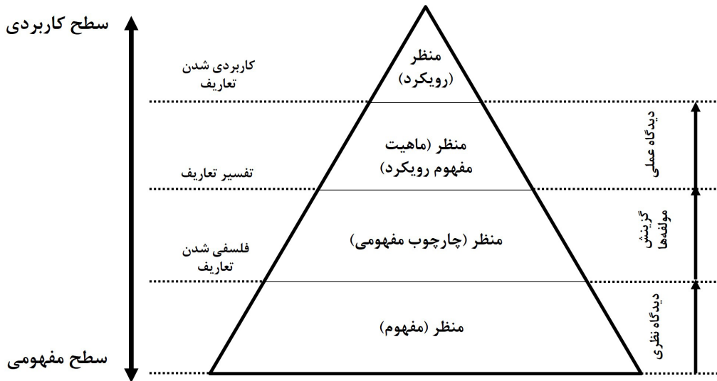
تصویر ۳. رویکرد منظر حاصل از کاربردی شدن چارچوب مفهومی منظر. مأخذ: نگارندگان.
