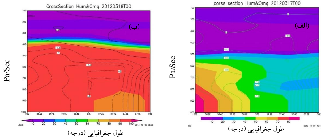
شکل ۲۴- نقشه سطح مقطع قائم رطوبت نسبی و سرعت قائم باد (بر حسب پاسکال بر ثانیه، ساعت ۰۰ UTC الف. روز ۲۰۱۲/۰۳/۱۷ ب. ۲۰۱۲/۰۳/۱۸)
