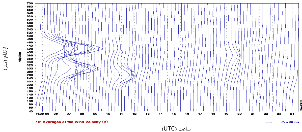
شکل ۱۱- پروفایل قائم تغییرات سرعت باد در روز ۲۰۱۲/۳/۱۱
