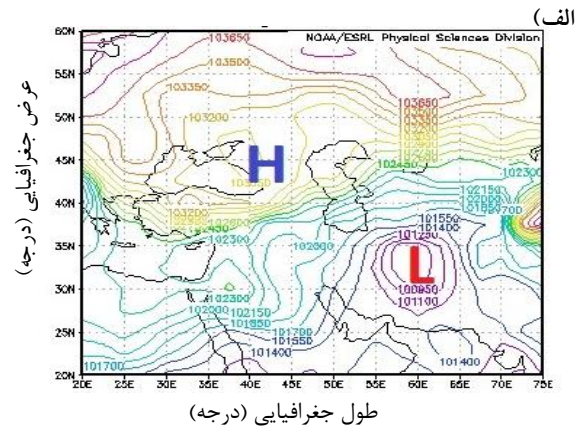
شکل ۲- نقشه سطح زمین تاریخ (الف) ۲۰۱۲/۰۲/۱۱ (ب) ۲۰۱۲/۰۲/۱۲ ساعت ۰۰ UTC
