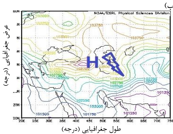
شکل ۲- نقشه سطح زمین تاریخ (الف) ۲۰۱۲/۰۲/۱۱ (ب) ۲۰۱۲/۰۲/۱۲ ساعت ۰۰ UTC
