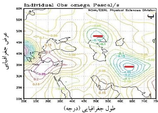
شکل ۳- (الف) نقشه تراز ۵۰۰ هکتوپاسکال (ب) سرعت قائم تراز ۵۰۰ هکتوپاسکال تاریخ ۲۰۱۲/۰۲/۱۱ ساعت ۰۰ UTC
