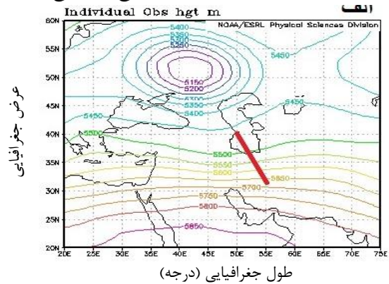
شکل ۳- (الف) نقشه تراز ۵۰۰ هکتوپاسکال (ب) سرعت قائم تراز ۵۰۰ هکتوپاسکال تاریخ ۲۰۱۲/۰۲/۱۱ ساعت ۰۰ UTC
