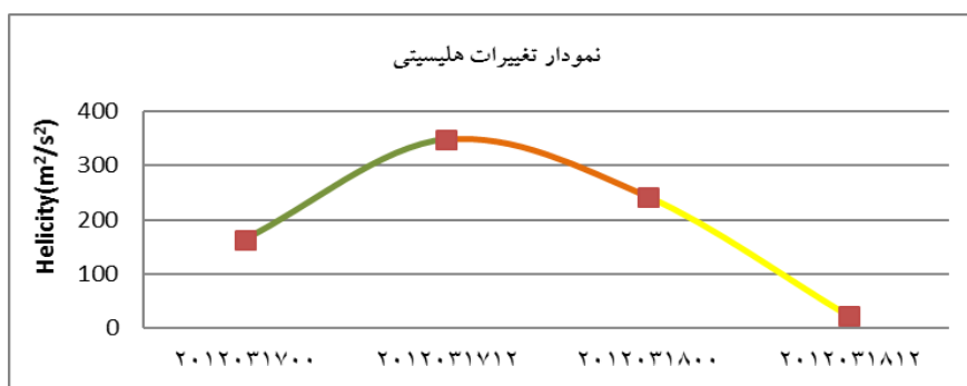
شکل ۲۲- نمودار تغییرات مقادیر هلیسیتی در طی ساعات وقوع رگبار برف تاریخ ۲۰۱۲/۰۳/۱۷
