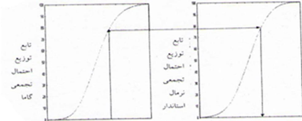
شکل ۲- طرح چگونگی تعیین شاخص SPI
