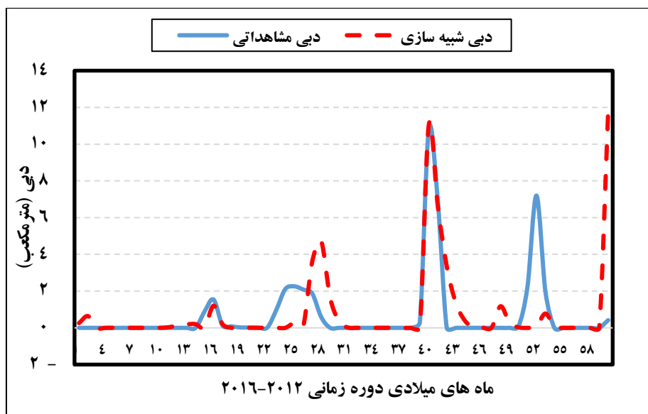
شکل ۵: مقایسه هیدروگراف‌های شبه‌سازی شده و مشاهداتی در دوره اعتبارسنجی ایستگاه خنداب
