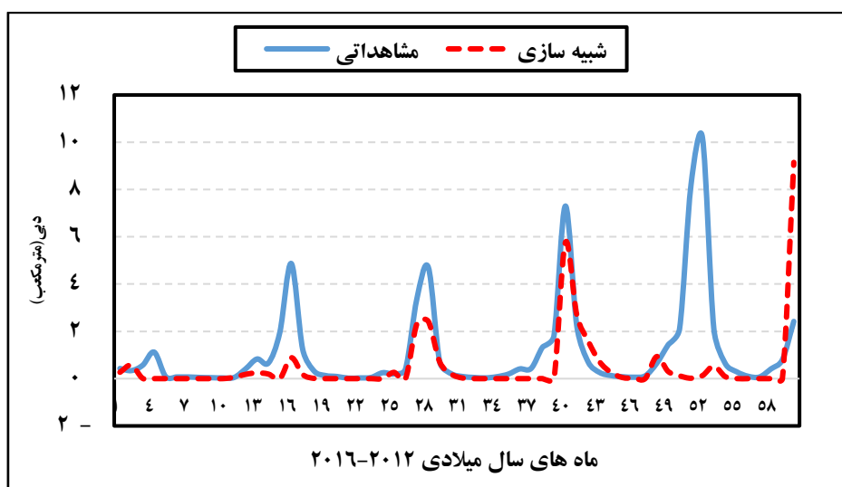
شکل ۶: مقایسه هیدروگراف‌های شبه‌سازی شده و مشاهداتی در دوره اعتبارسنجی ایستگاه پل دوآب
