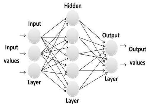
شکل ۲. شماتیک MLP
