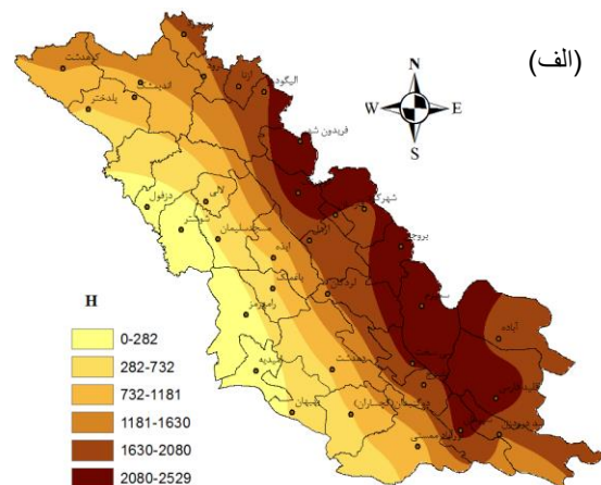
شکل ۳: الف) تغییرات ارتفاعی ایستگاه‌های مورد مطالعه، ب) نقشه هم‌دمای منطقه مورد مطالعه بر اساس میانگین دمای سالانه
