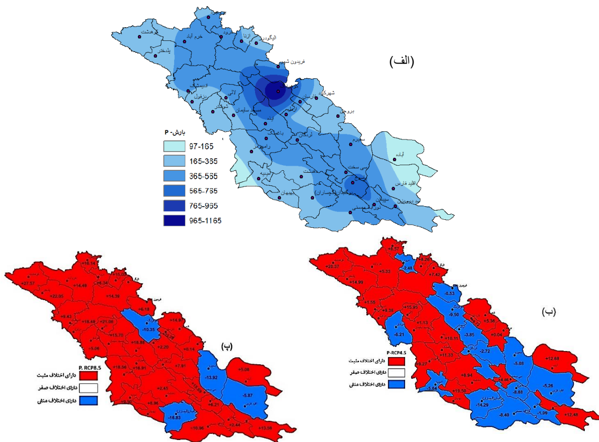
شکل ۵: الف) نقشه هم‌بارش منطقه مورد مطالعه بر اساس میانگین بارش سالانه در دوره تاریخی (ب) تغییرات بارش سالانه در سناریوی RCP4.5 نسبت به دوره تاریخی، (پ) تغییرات بارش سالانه در سناریوی RCP8.5 نسبت به دوره تاریخی
