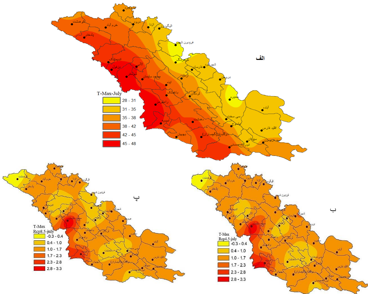
شکل ۹: الف) نقشه هم‌دمای منطقه مورد مطالعه بر اساس میانگین دمای بیشینه ژولای در دوره تاریخی ب) تغییرات میانگین دمای بیشینه ژولای در سناریوی RCP4.5 نسبت به دوره تاریخی، پ) تغییرات میانگین دمای بیشینه ژولای در سناریوی RCP8.5 نسبت به دوره تاریخی
