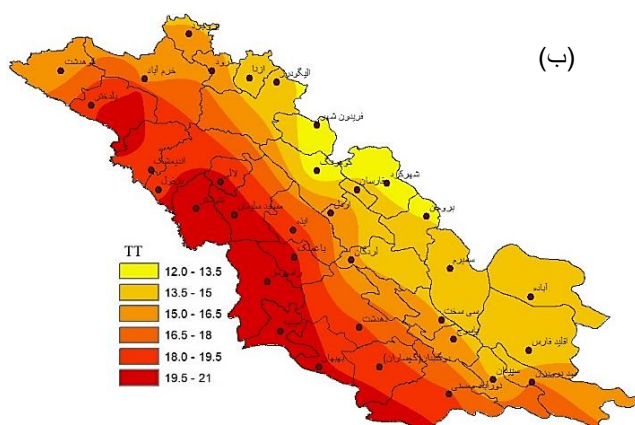
شکل ۳: الف) تغییرات ارتفاعی ایستگاه‌های مورد مطالعه، ب) نقشه هم‌دمای منطقه مورد مطالعه بر اساس میانگین دمای سالانه
