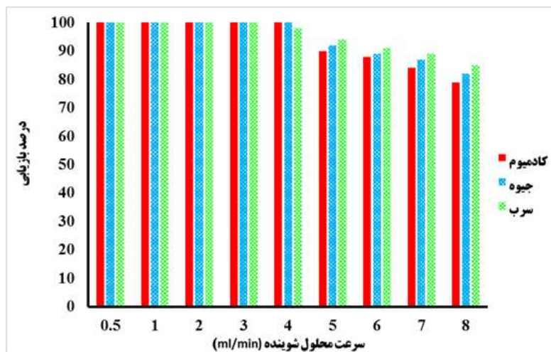
شکل ۹- اثر سرعت جریان محلول شوینده بر روی بازایی
