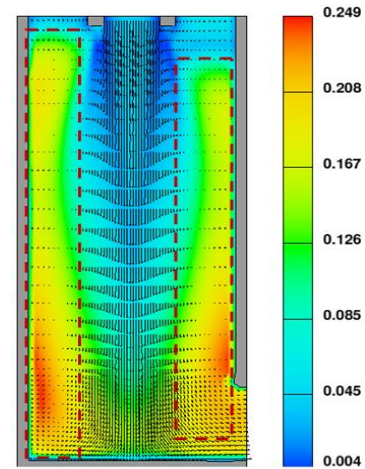
شکل (۱۳) عدم تقارن در ابعاد گردابه‌های تشکیل شده در طرفین جت ورودی
