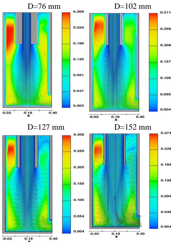
شکل (۷) طول مقیاس آشفتگی برای قطر مختلف لوله ورودی D=76 mm D=102 mm
