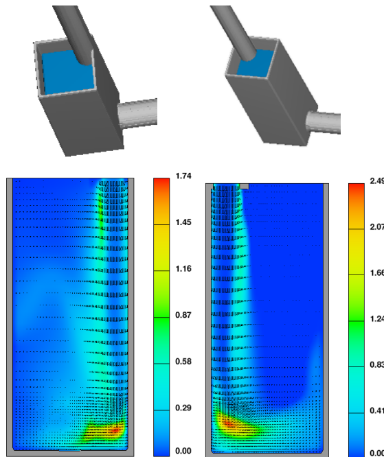
شکل (۱۴) نتایج اتلاف انرژی در موقعیت‌های مختلف جت ورودی به اتاقک اتلاف
