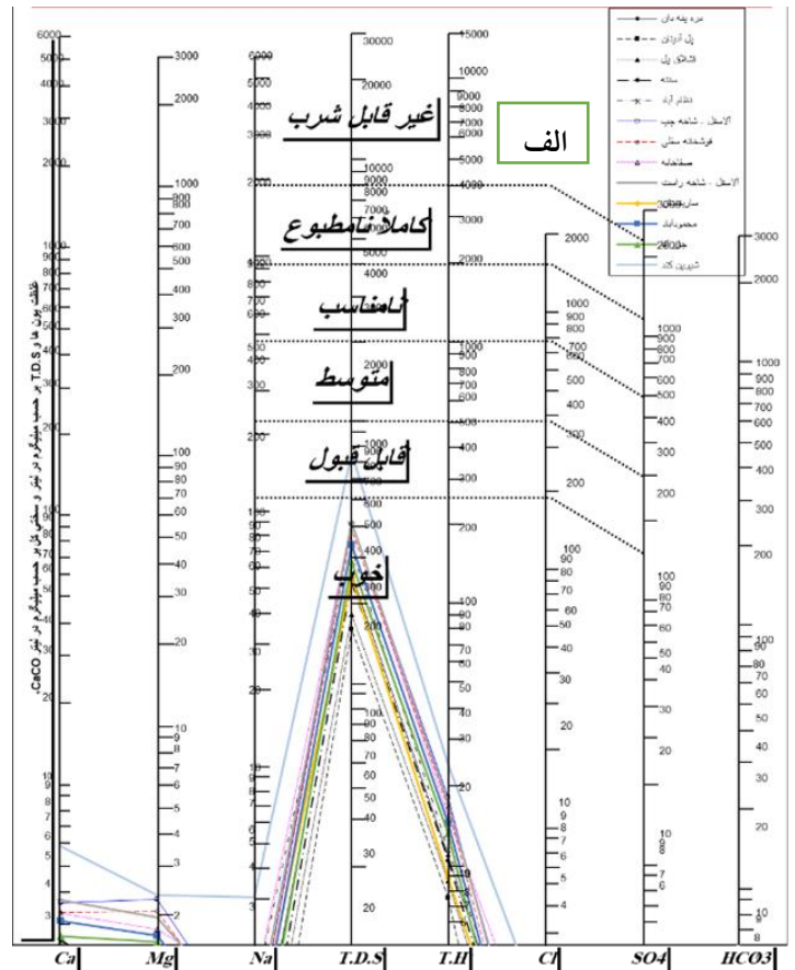
شکل (۳). کیفیت آب در دیاگرام شولر الف) زرينه رود، ب) سيمينه رود
