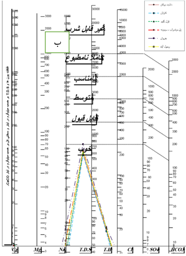
شکل (۳). کیفیت آب در دیاگرام شولر الف) زرينه رود، ب) سيمينه رود
