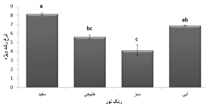
شکل ۲. مقایسه داده‌های (میانگین \pm انحراف معیار) تغییرات نرخ رشد ویژه بین تیمارهای مختلف. (حروف انگلیسی متفاوت بیان گر وجود اختلاف معنی‌دار بین تیمارها در سطح ۰/۰۵ می‌باشد).
