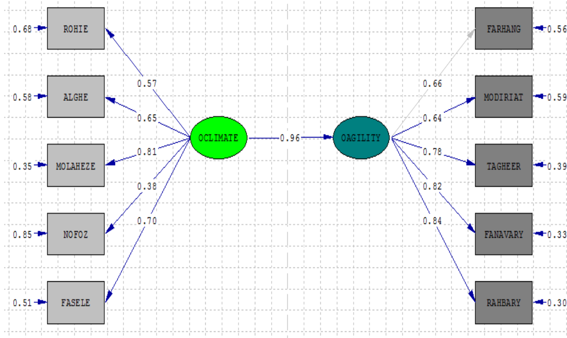
شکل ۳. مدل اثر کلی جو سازمانی بر چابکی سازمانی وزارت ورزش و جوانان در حالت ضریب اثر (Standard Solution)
